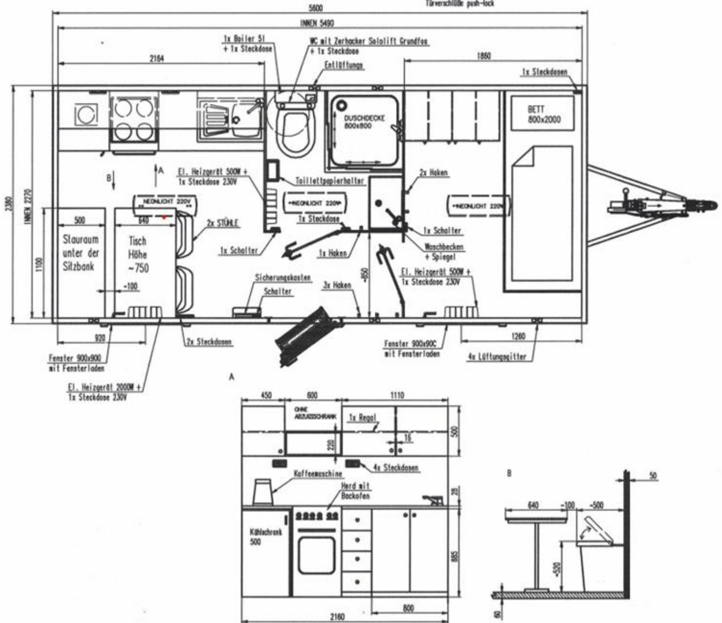
Mobi 5644, 2 Plätze, Doppelbett, Wassertoilette, Dusche, Küche, Garderobe
