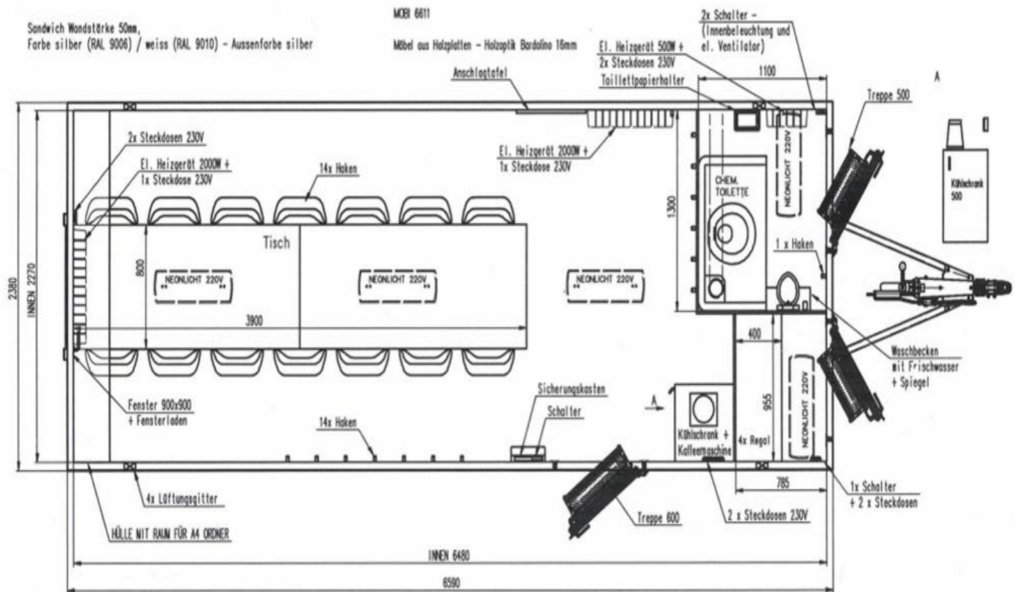
Mobi 6611, 14 Plätze, Chemische Toilette, Werkzeugraum
