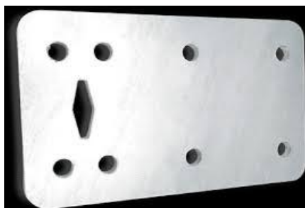
Befestigungsplatte für Kurbelstützen Stahl feuerverzinkt. Länge 220mm, Breite 134mm, Dicke 8mm. Lochmass 80 x 80mm, 30 x 80mm Lochgrösse 13mm Für Böckmann Kipper Miet-Lift Art. Nr. 52250
