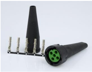
Aspöck Bajonett-Verbinder rechts mit 2 poligem Abgang für Kennzeichenkabel DIN ISO 1724 Miet-Lift Art.Nr. 54791
