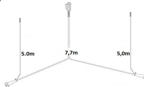
Kabel mit 13-poligem Stecker und Bajonettstecker, 1 x gelb, 1 x grün, Bajonettstecker 8-polig 7,7m Kabellänge, 2 x Abgang 5.0 Miet-Lift Art.Nr. 54815
