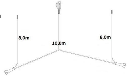
Kabel mit 13-poligem Stecker und Bajonettstecker, 1 x gelb, 1 x grün, Bajonettstecker 5-polig 10m Kabellänge, 2 x Abgang 8.0m Miet-Lift Art.Nr. 54813
