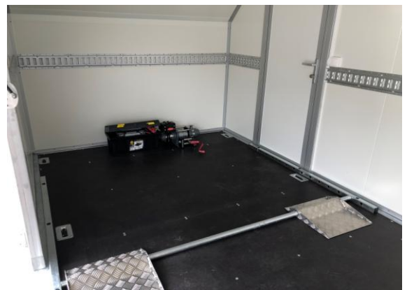
Radanschlag seitlich und in der Länge verstellbar
