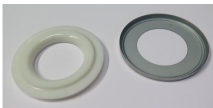
Lagerdichtring / Wellendichtring 2-teilig Kunststoffscheibe mit Metallkappe. BPW / Peitz zu S2005-5. 35 x 62 x 8mm. BPW 03.120.43.05.0
