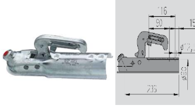
Kugelpkupplung AK 7 Ausführung B Gesamtgewicht 750/800kg Anschluss 60mm rund Miet-Lift Art. Nr. 51001
