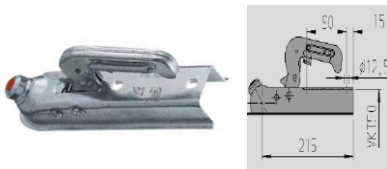
Kugelpkupplung AK 7 Ausführung D Gesamtgewicht 750/800kg Anschluss 50mm vierkant Miet-Lift Art. Nr. 51004
