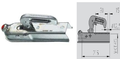
Kugelpkupplung AK 7 Ausführung G Gesamtgewicht 750/800kg Anschluss 45mm vierkant Miet-Lift Art. Nr. 51003
