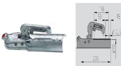
Kugelpkupplung AK 7 Ausführung C Gesamtgewicht 750/800kg Anschluss 70mm rund Miet-Lift Art. Nr. 51002
