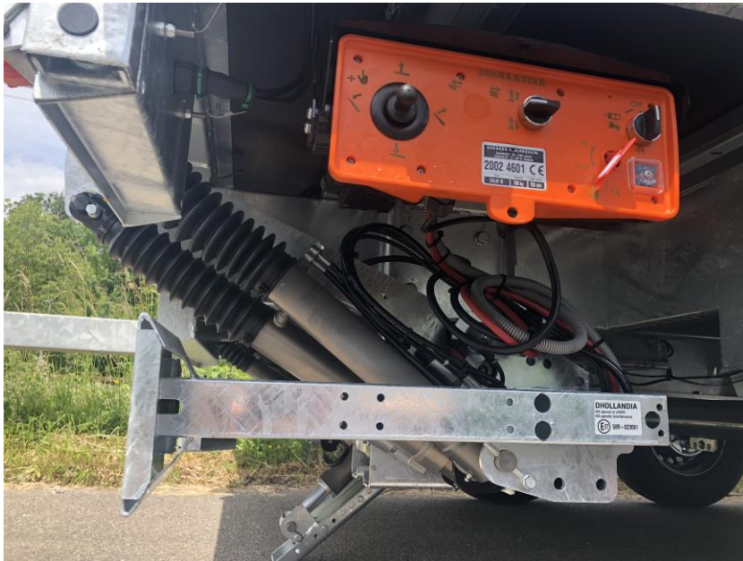
Steuerkasten Hebebühne mit Stromunterbruch-Schalter, abschliessbar
