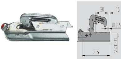
Kugelkupplung AK 7 Ausführung G Gesamtgewicht 750/800kg Anschluss 45mm vierkant Miet-Lift Art. Nr. 51003
