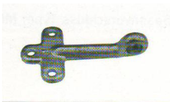
Einfall-Oese Grösse I Totallänge 125mm, Lochabstand 50/33mm Miet-Lift Art.Nr. 55173
